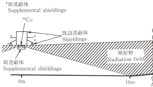
第3図 遮蔽体設置後のガンマーフィールドの照射野 Fig. 3. Radiation field of the Gamma Field after the installation of the shielding.
