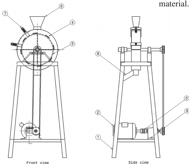
Fig. 3. Arecanut dehusker
