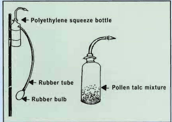
Fig. 27. Pole pollination device
